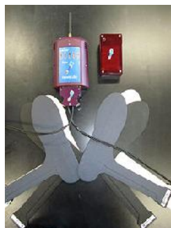
شکل ۱: سیستم اندازه گیری فشار کف پای پدار
